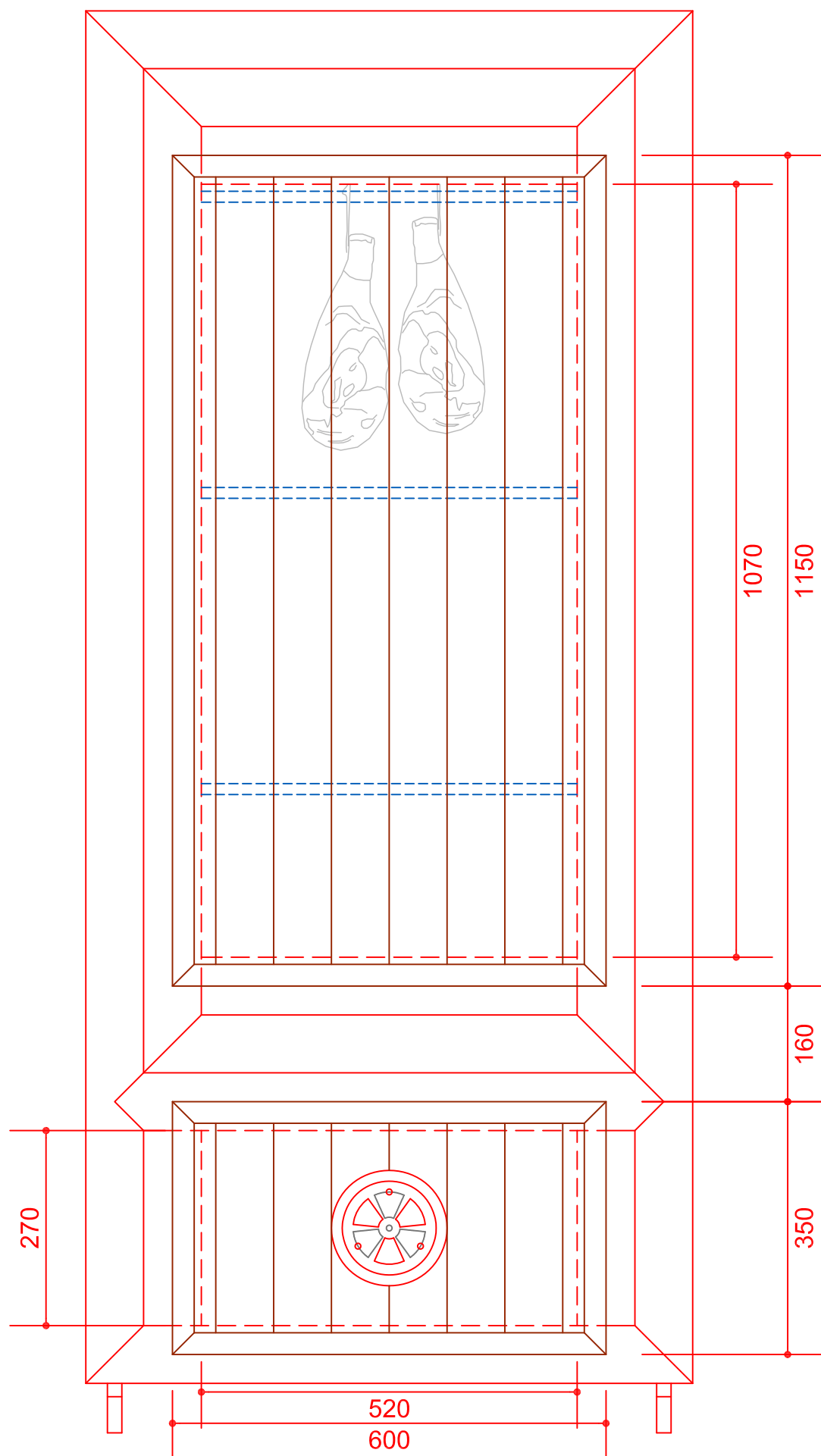
Vorderansicht (geschlossen)
